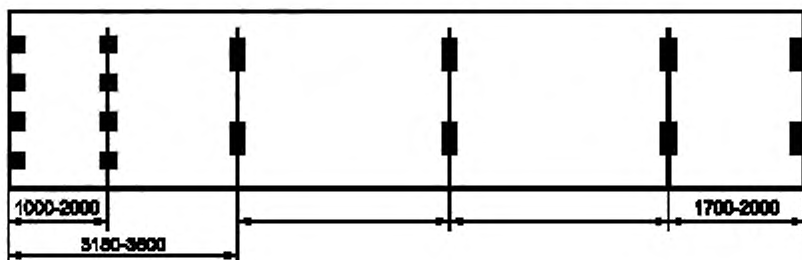
Рисунок В.8* — Размещение шести пар опорных (контактных) площадок (одна пара на каждый торец плюс четыре промежуточные пары)
