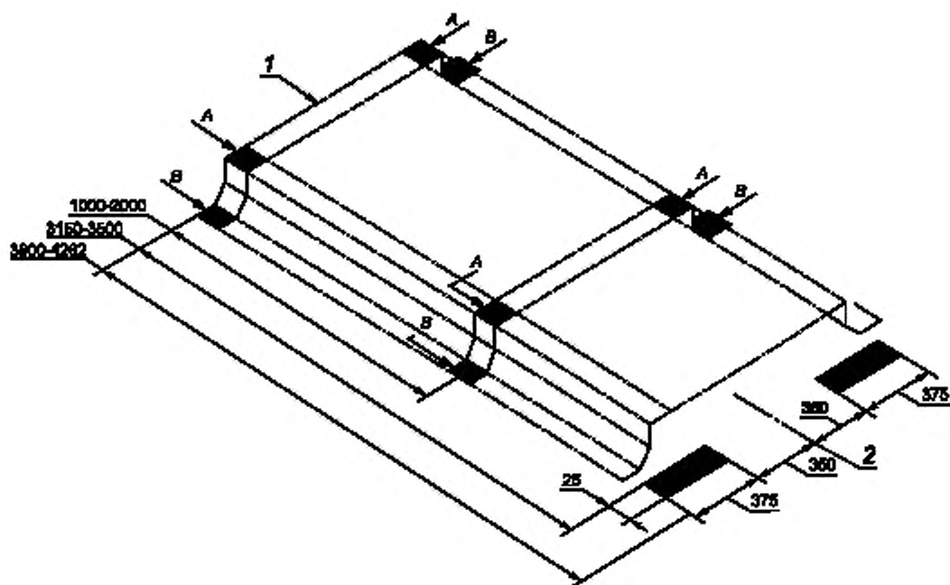
Рисунок В.9 — размещение семи пар опорных (контактных) площадок
