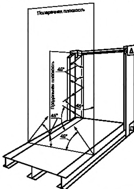
Рисунок Ф.1 — Устройство для крепления груза — варианты приложения испытательной нагрузки
