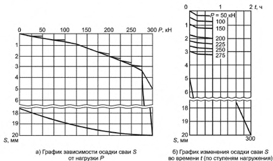
Рисунок К.2 — Графики результатов испытаний грунтов эталонной свай и свай-зондом на вдавливающую нагрузку
