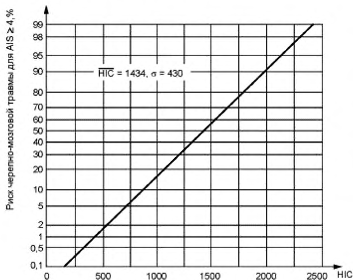
Рисунок А.3 — Риск черепно-мозговой травмы для AIS \geq 4 , как функция HIC при длительности удара 15 мс
