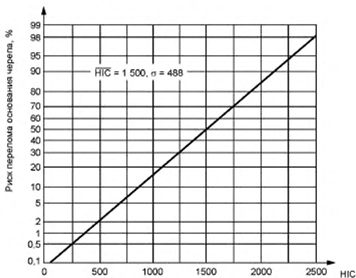
Рисунок А.1 — Риск перелома основания черепа для AIS \geq 2 , как функция НИС при длительности удара 15 мс
