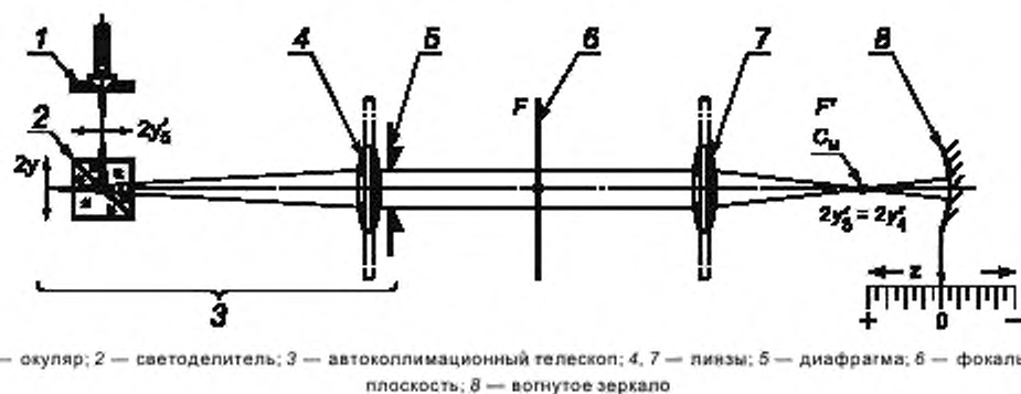
Рисунок А.1 — Установка для проверки пробной очковой линзы
