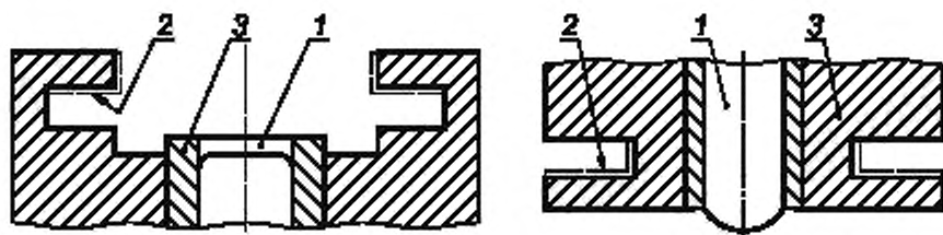
1 — часть P ; 2 — часть Q ; 3 — изоляция
