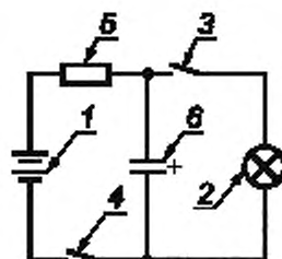
1 — батарея; 2 — лампа-вспышка; 3 — выключатель синхронизатора; 4 — выключатель; 5 — резистор; 6 — триггерный конденсатор
