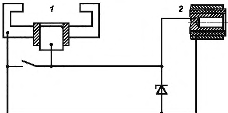
1 — колодка; 2 — гнездо (розетка)
