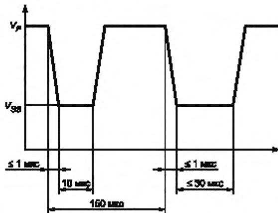
Рисунок А.2 — Форма сигнала напряжения на выводах цепи поджига блока фотовспышки со схемой подавления помех
