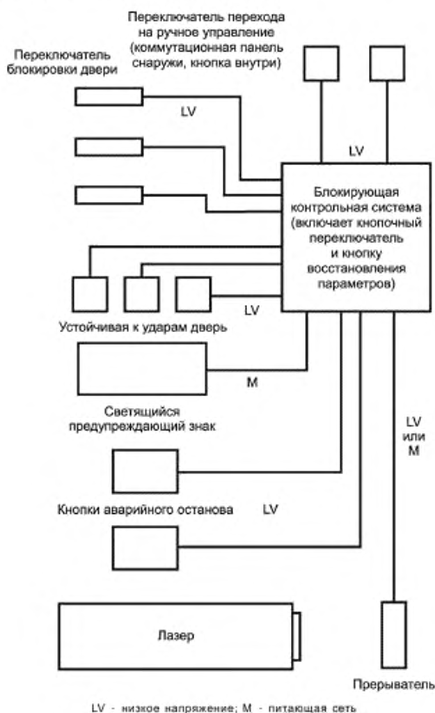
Рисунок А.3 — Система блокировки с запиранием
