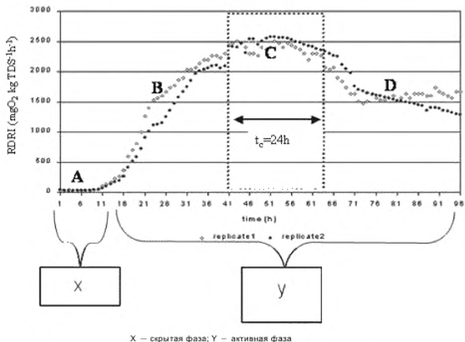
Рисунок А.1 — Линия испытания RDRl в зависимости от времени
