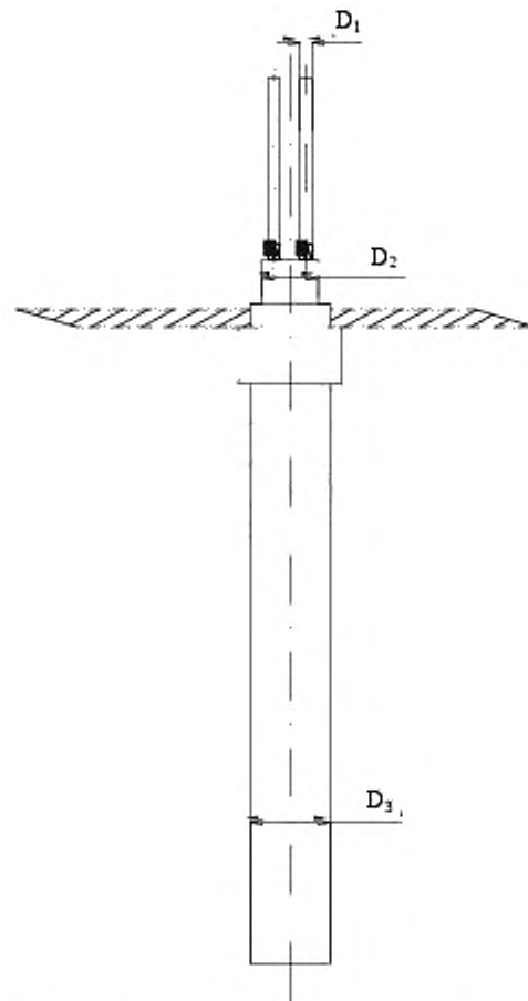
Рисунок 8 – Испытательное устройство для испытания на распространение огня
