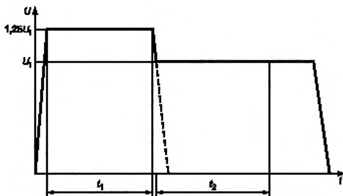
Рисунок 3 – Испытательное напряжение
