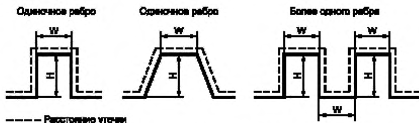
Рисунок 2 — Размеры высоты ( H ) и ширины ( W ) ребер
