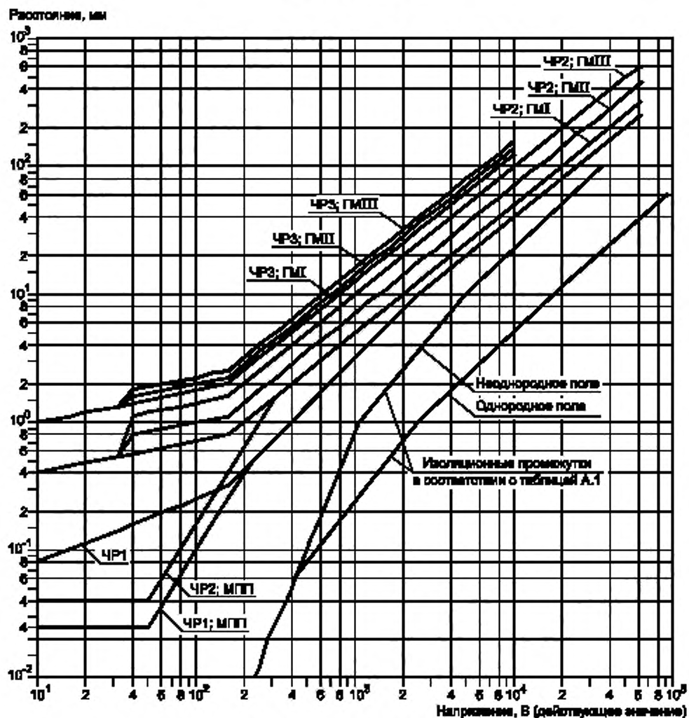
Рисунок E.1 — Взаимосвязь между расстояниями утечки, указанными в таблице F.4 и изоляционными промежутками из таблицы A.1
