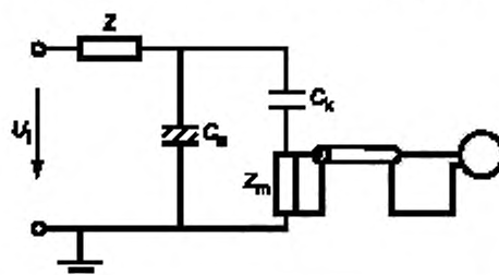
Рисунок С.1 — Заземленный испытательный образец
