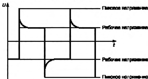
Рисунок 1 — Повторяющееся пиковое напряжение
