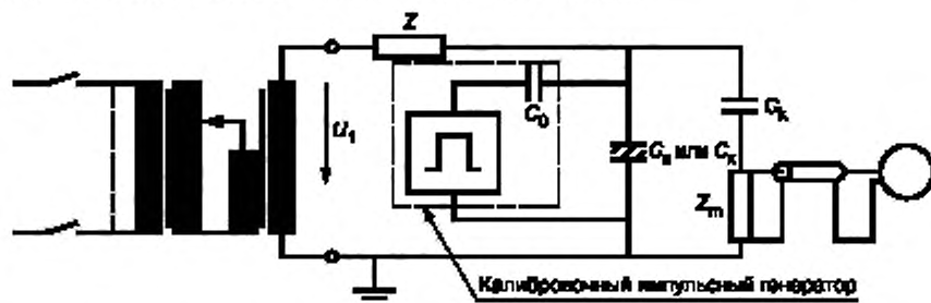
Рисунок С.3 — Калибровочная цепь для заземленного испытуемого образца
