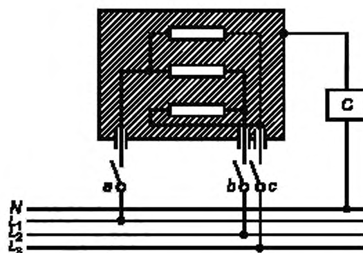
С - схема из IEC 60990 (рисунок 4); L_1, L_2, L_3, N - питание с нейтральным проводом
