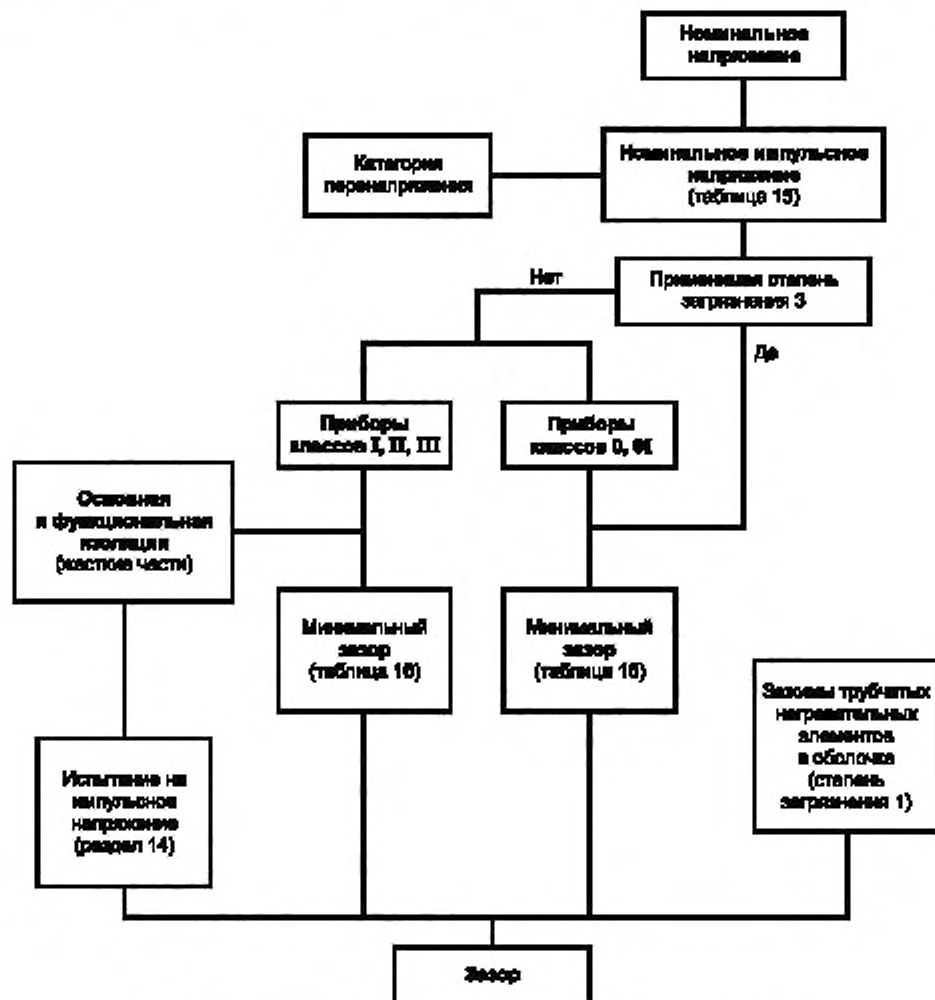
Рисунок L.1 – Последовательность для определения зазоров
