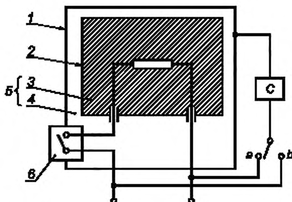
Рисунок 1 – Схема измерения тока утечки при рабочей температуре для однофазных приборов класса II
