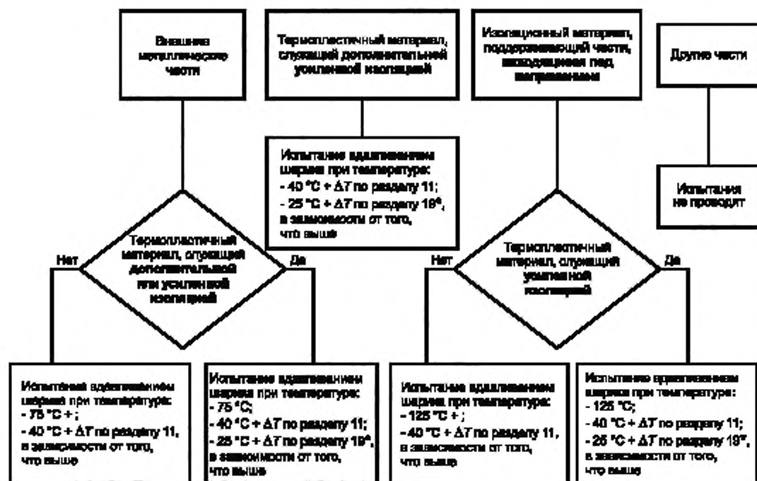
Рисунок О.1 – Испытания на теплостойкость
