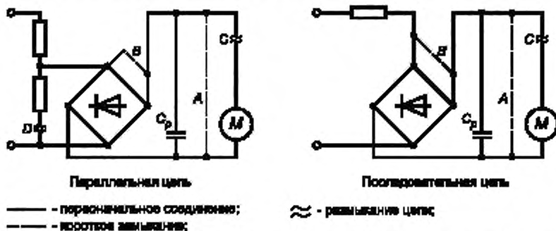
Рисунок I.1 – Имитация условий неисправности
