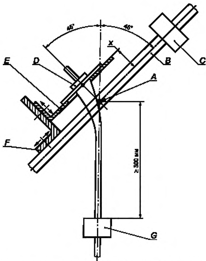
А – ось качания; В – качающийся элемент (рама); С – противовес; D – образец; E – регулируемая несущая плата. F – регулируемый кронштейн, G – груз
