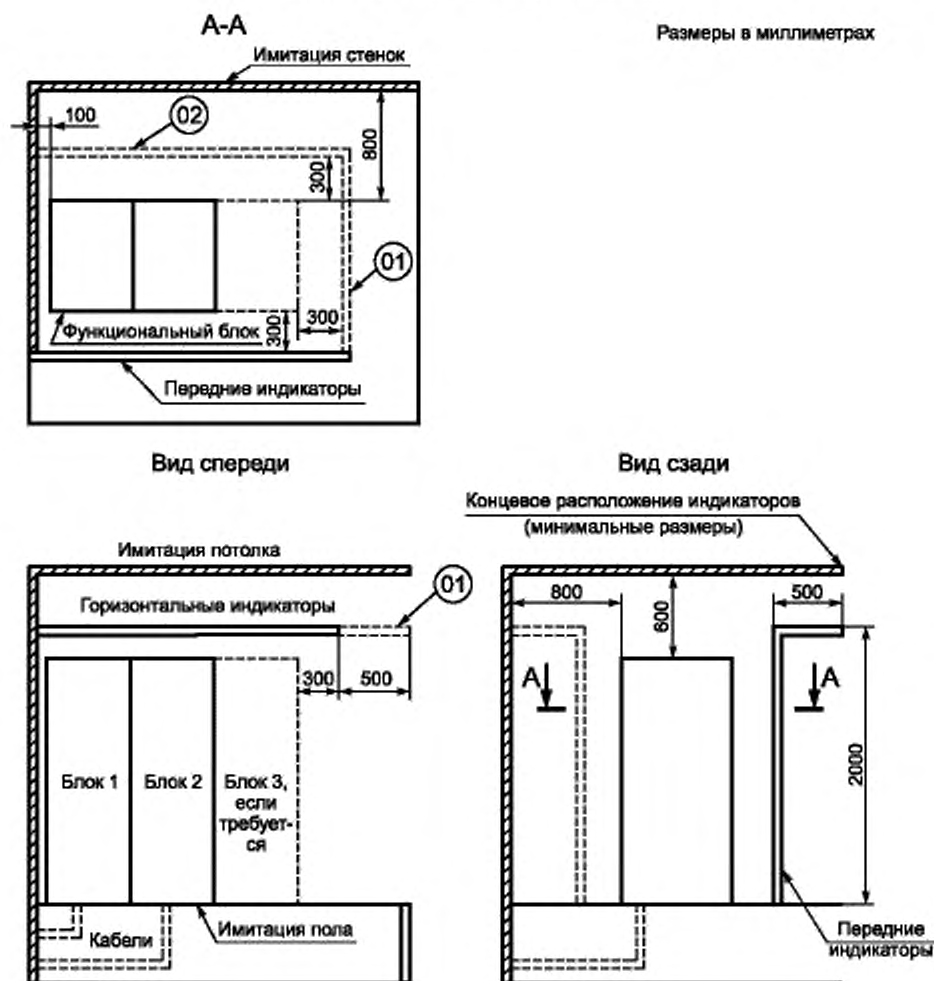
Рисунок А.3 — Положение индикаторов
