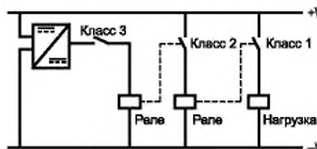
Рисунок 1 — Примеры классов контактов
