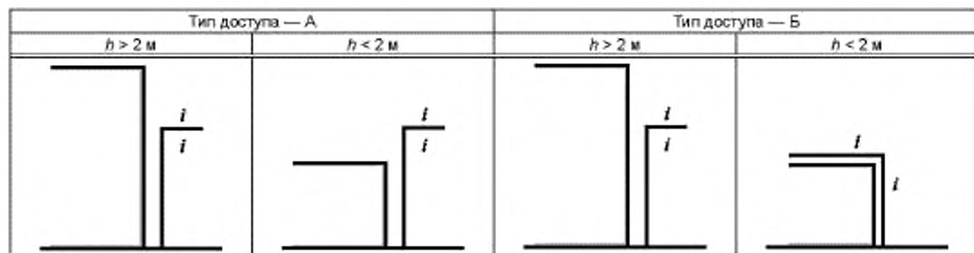
Рисунок А.3 — Положение индикаторов
