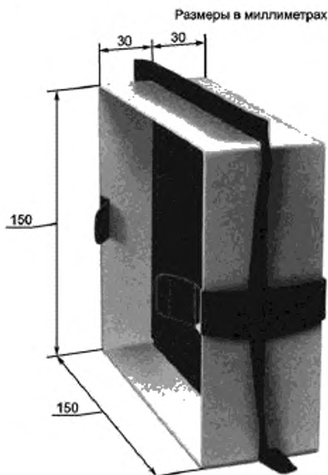
Рисунок А.1 — Монтажная рамка для вертикального индикатора
