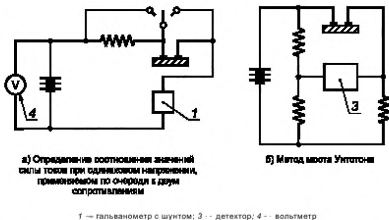
Рисунок Б.3 — Схема для измерения сопротивления электрической изоляции сравнительным методом
