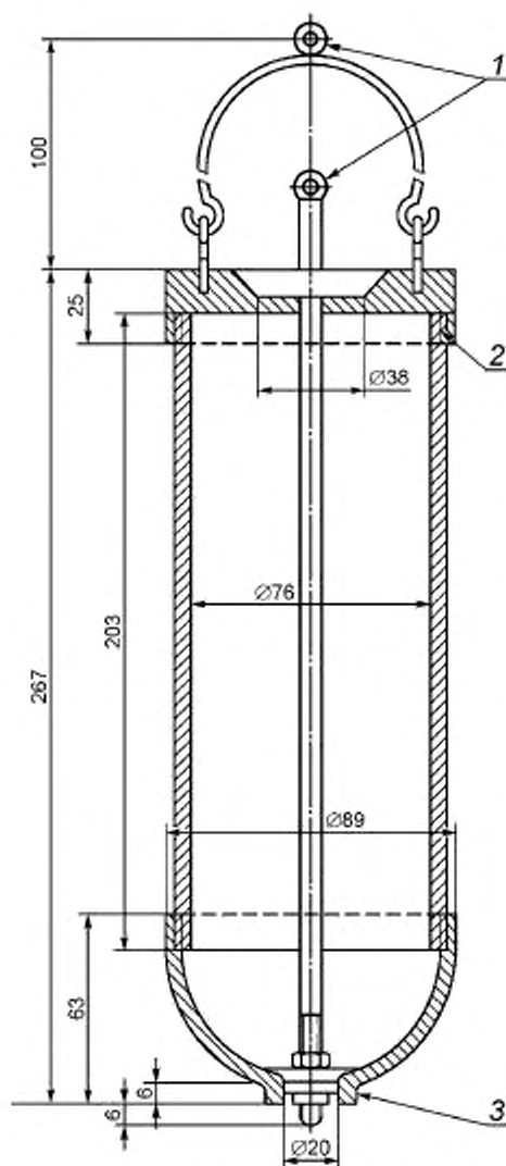
Рисунок 1 — Глубинный пробоотборник
