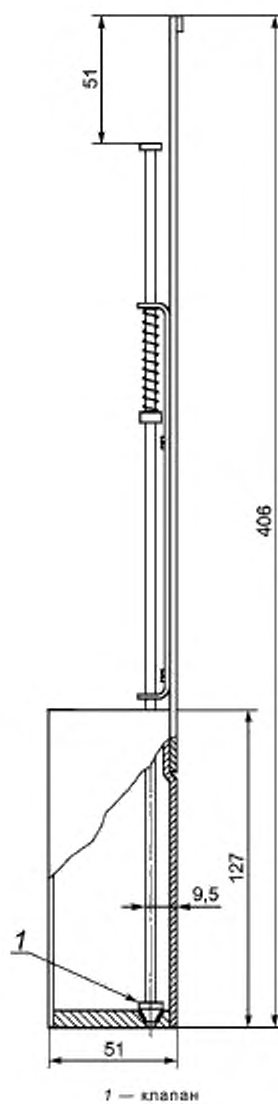
Рисунок 2 — Поверхностный пробоотборник
