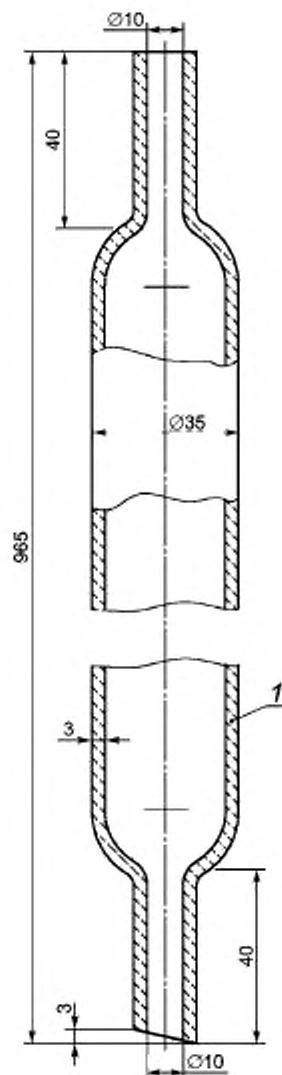
Рисунок 3 — Пипетка
