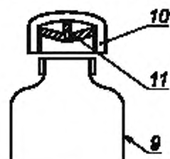
б — Пример уплотнения крышки для бутылки
