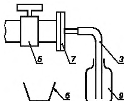
а — Проверка отбора проб в бутылки
