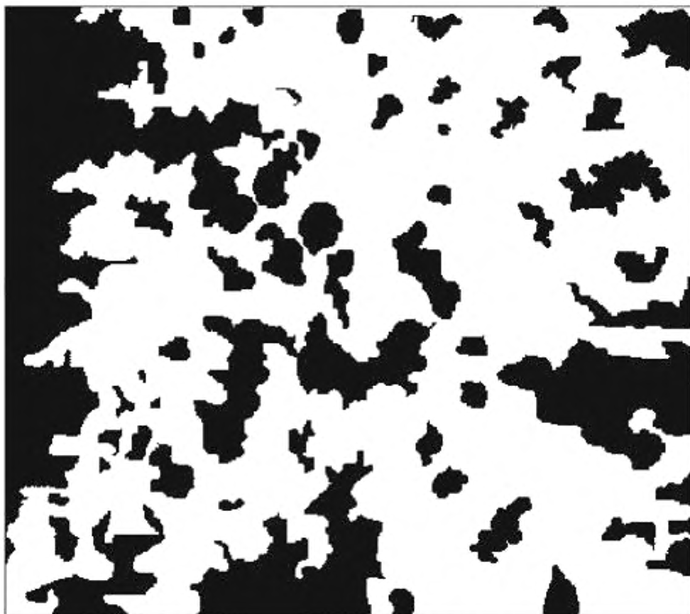
Рисунок Ж.5 — Коррозия металла, балл K5 (или R/5)
