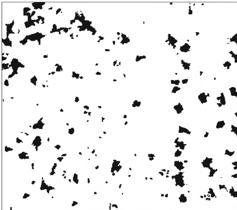
Рисунок Ж.4 — Коррозия металла, балл K4 (или R4)
