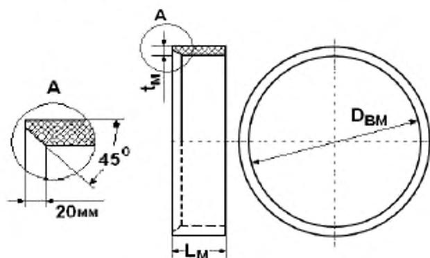
Рисунок 4.6 – Основные размеры соединительных муфт для сегментов трубопроводов типа К
