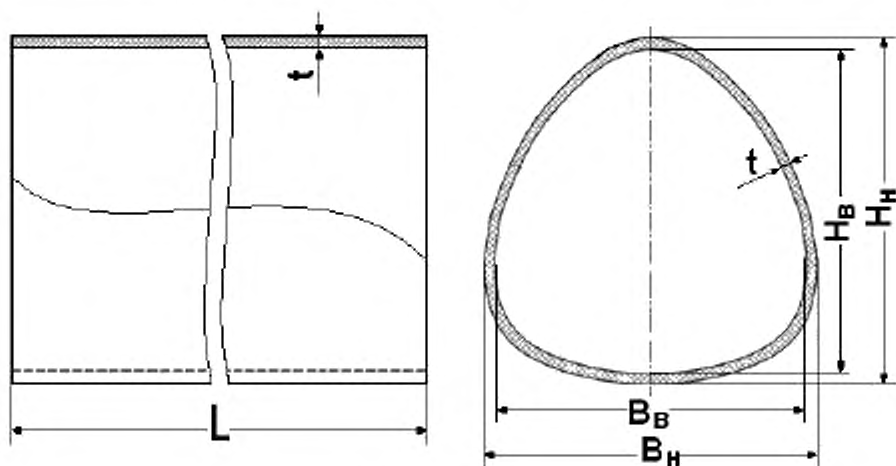
Рисунок 4.1 – Основные размеры сегментов трубопроводов типа К
