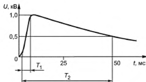
Рисунок 6 — Импульс высокого напряжения
