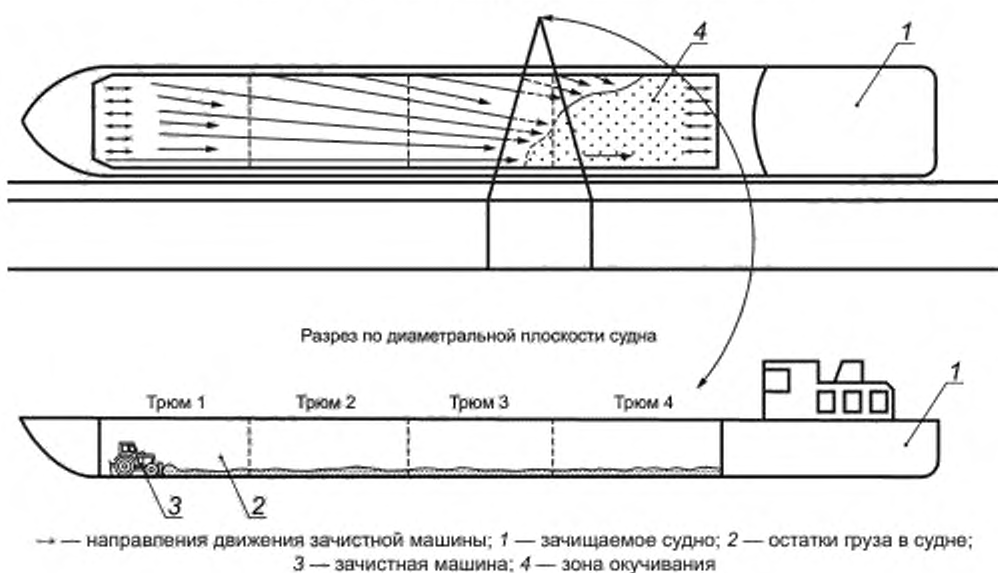
Рисунок 2 — Схема использования зачистной машины
