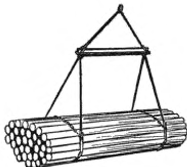
Рисунок 7 — Схема строповки длинномерного груза
