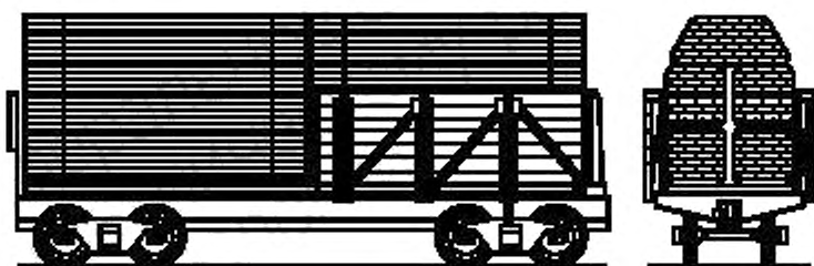
Рисунок 11 — Схема размещения груза в полувагоне
