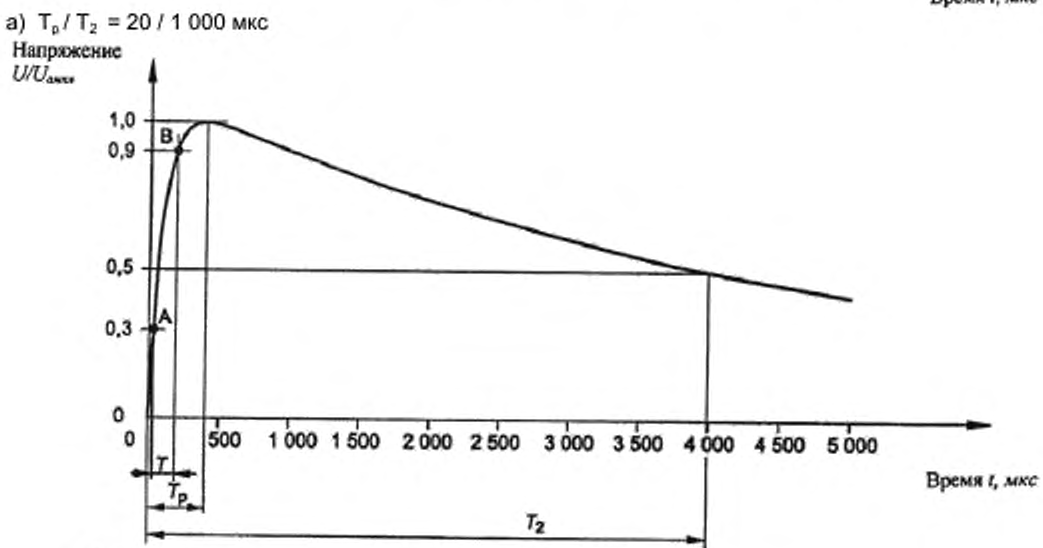
Рисунок 3 - Аperiodический коммутационный импульс
