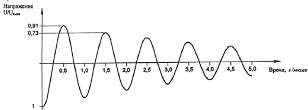
Рисунок 5 - Затухающее переменное напряжение ( f_r = 1 кГц, D_r = 0,2 )
