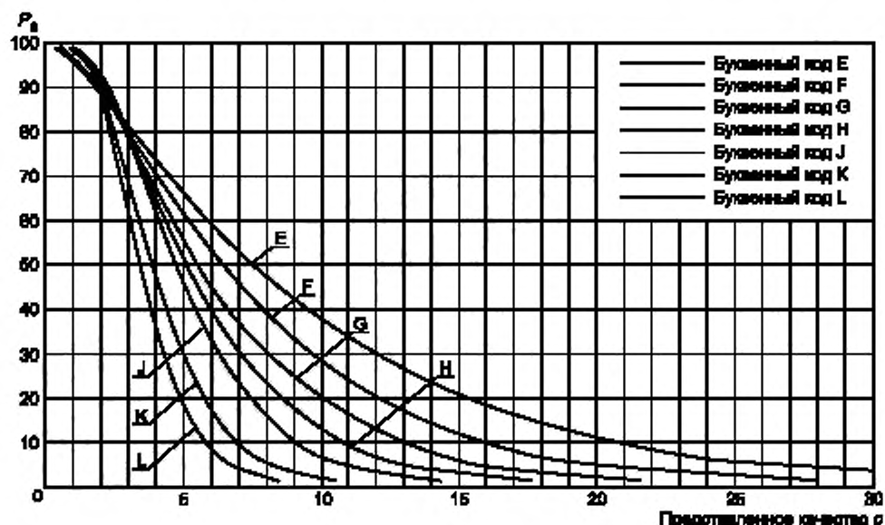
Рисунок 9 — Кривые OC (PX) для сокращенного контроля, AQL (ППК) = 1,0
