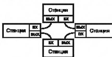
Рисунок 4 — Топология «кольцо»
