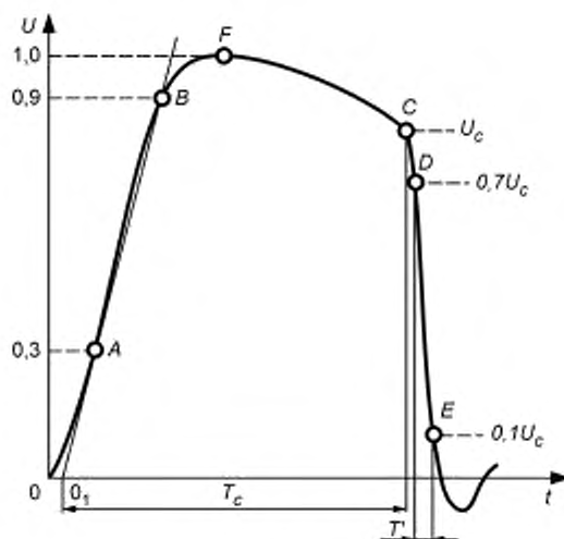
Рисунок 12 — Грозовой импульс, срезанный на спаде импульса
