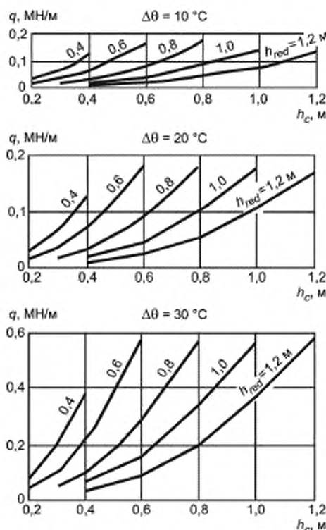
Рисунок 40 — График значений нагрузки q
