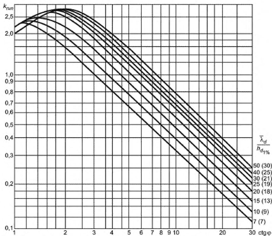
Рисунок 10 — Графики значений коэффициента k_{ум}
