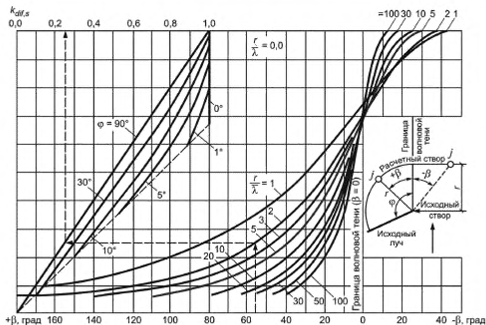
Рисунок А.7 — Графики для определения значений коэффициента k_{диф,s}
