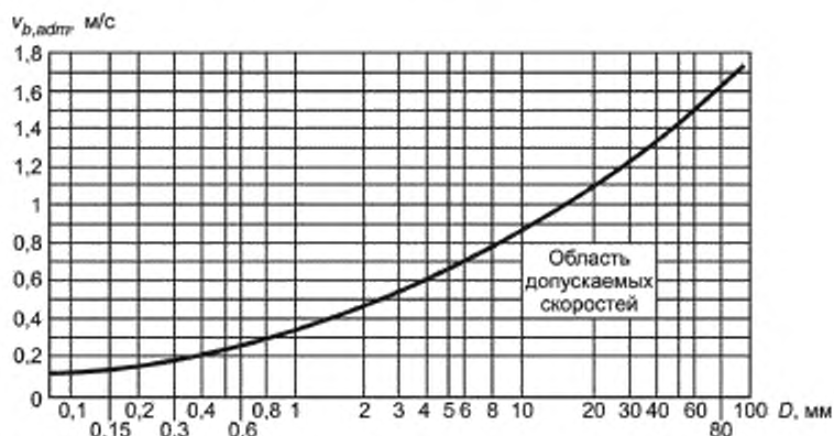
Рисунок 7 — График допустимых значений неразрывающих донных скоростей
