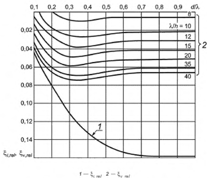
Рисунок 21 — Графики значений относительных ординат
