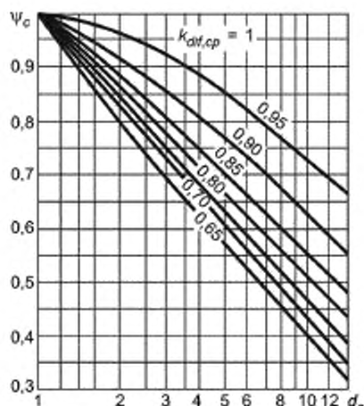
Рисунок А.8 — Графики значений коэффициента \psi_c
