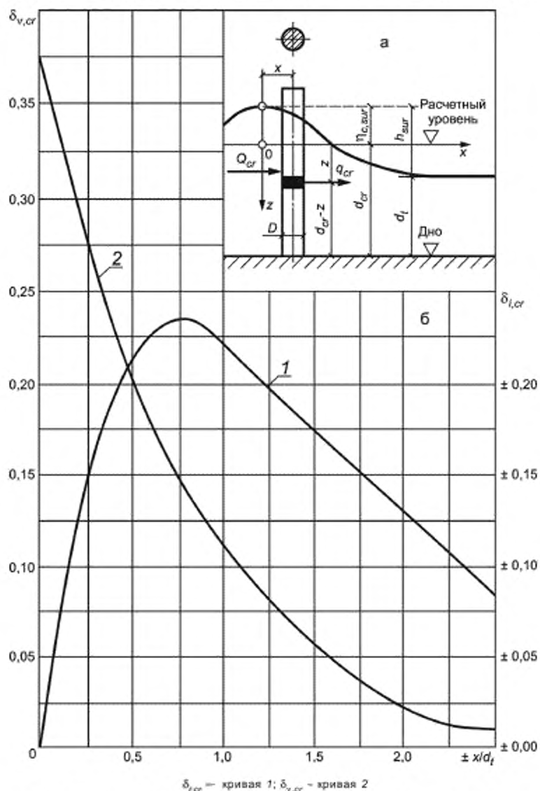
Рисунок 24 — Схема к определению нагрузок от разбивающихся волн и графики значений коэффициентов \delta_{l,cr} и \delta_{v,cr}
