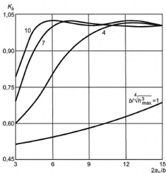
Рисунок 44 — Графики значений коэффициента K_k
