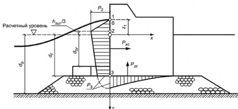
Рисунок 8 — Эюры давления разбивающихся волн на вертикальную стену
