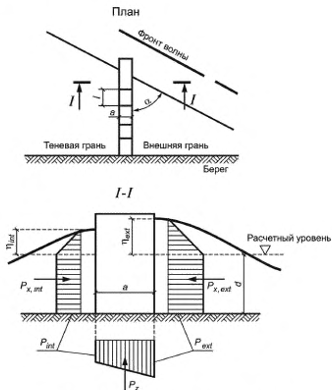
Рисунок 30 — Эпюры волнового давления на буня
