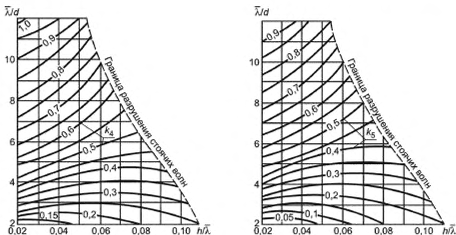
Рисунок 4 — Графики значений коэффициентов k_4 и k_5
