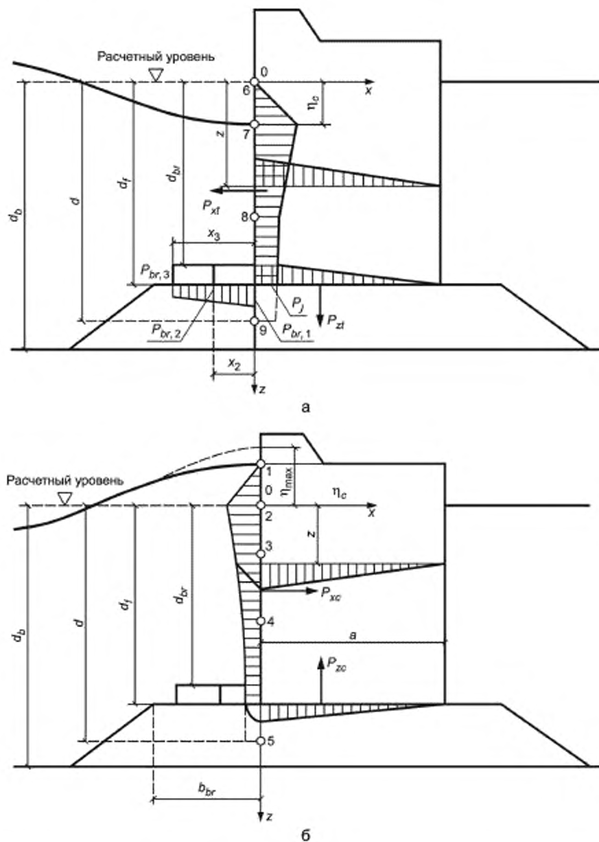
Рисунок 1 — Эпюры давления стоячих волн на вертикальную стену со стороны открытой акватории
