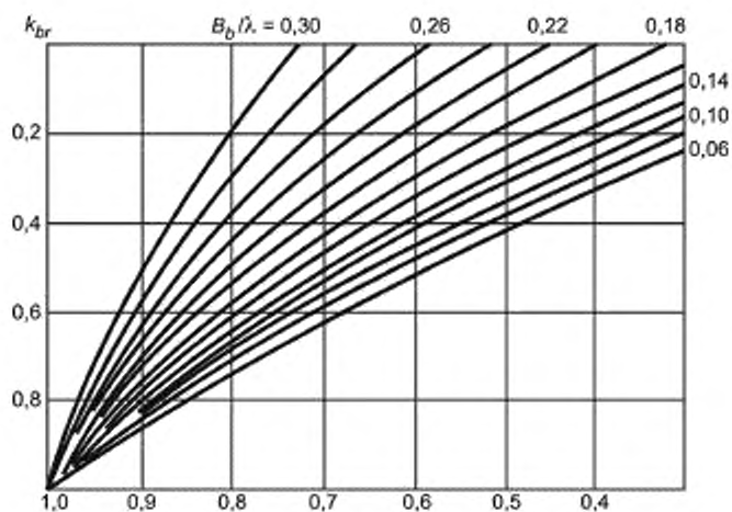
Рисунок 2 — Графики значения коэффициента k_{br}
