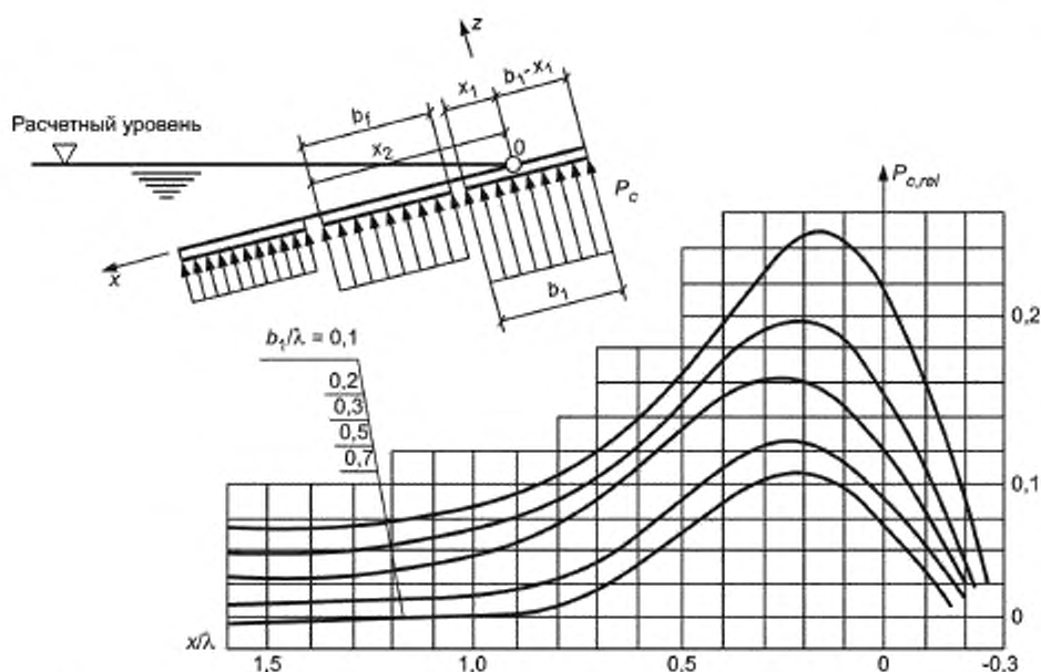
Рисунок 12 — Графики для определения относительного волнового противодавления
