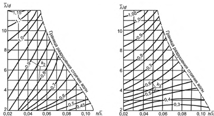
Рисунок 3 — Графики значений коэффициентов k_2 и k_3
