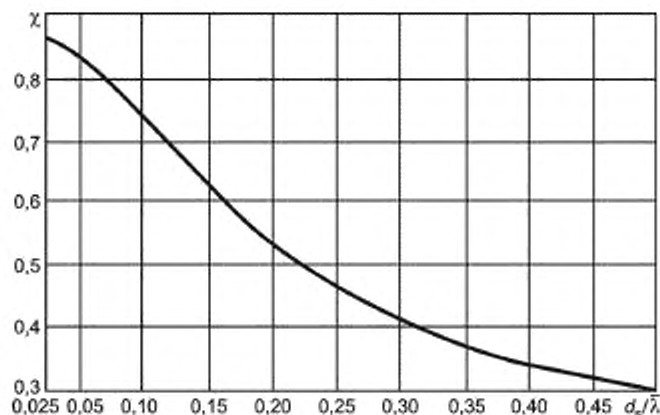
Рисунок 32 — График значений коэффициента \chi
