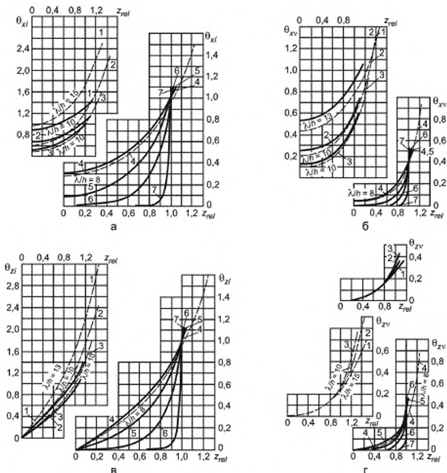
Рисунок 19 — Графики коэффициентов линейной нагрузки от волн \theta_{xi} , \theta_{xv} , \theta_{zi} , \theta_{zv} , при d/\lambda : 1—0,1; 2—0,15; 3—0,2; 4—0,3; 5—0,5; 6—1; 7—5 и \lambda/h = 40 — сплошные линии; \lambda/h = 8, 10, 13, 15 — штриховые линии
