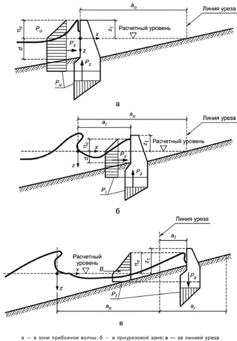
Рисунок 27 — Эпюры волнового давления на вертикальную волнозащитную стену при расположении сооружения
