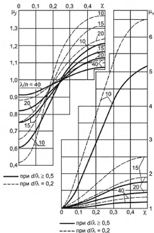
Рисунок 22 — Графики значений инерционного \mu_i и скоростного \mu_v коэффициентов фазы
