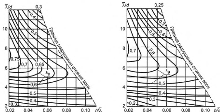
Рисунок 5 — Графики значений коэффициентов k_8 и k_9
