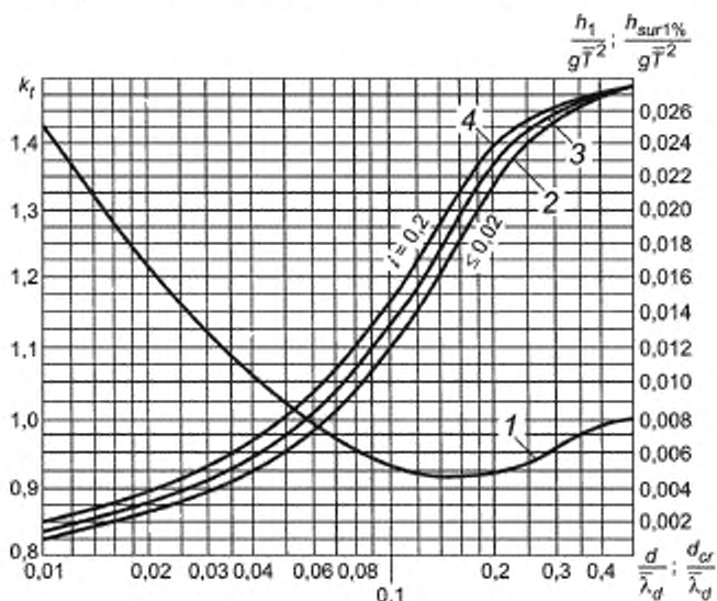
Рисунок А.5 — Графики для определения 1 — коэффициента k_r ; 2, 3 и 4 — величин d_{cr}/\bar{\lambda}_d
