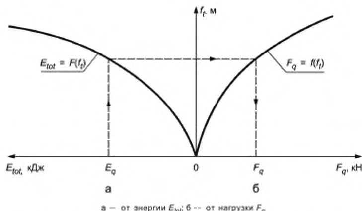
Рисунок 33 — Схема построения графиков зависимости деформаций отбойного устройства (и причального сооружения) f_c
