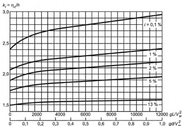
Рисунок А.2 — Графики значений коэффициента k_i
