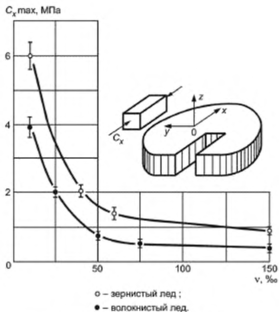
Рисунок Б.3 — Зависимость максимального предела прочности морского льда при одноосном сжатии от количества жидкой фазы
