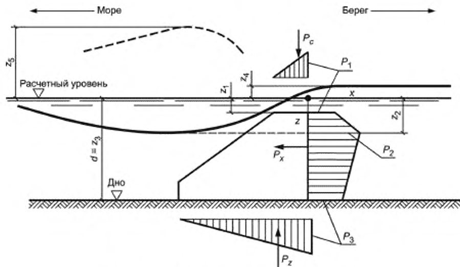
Рисунок 26 — Эпюры волнового давления на подводный волнолом
