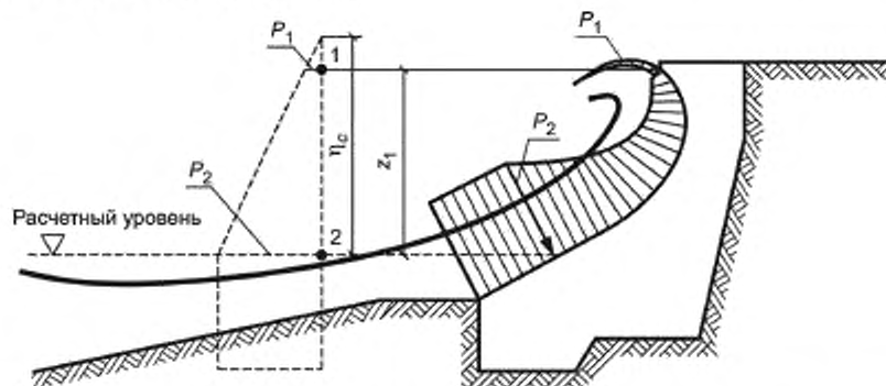
Рисунок 29 — Эпюра давления волн на криволинейный участок волнозащитной стены
