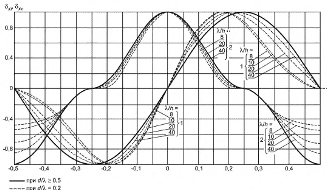
Рисунок 18 — Графики значений коэффициентов сочетания инерционного \delta_x (график 1) и скоростного \delta_v (график 2) компонентов горизонтальной линейной нагрузки от волн
