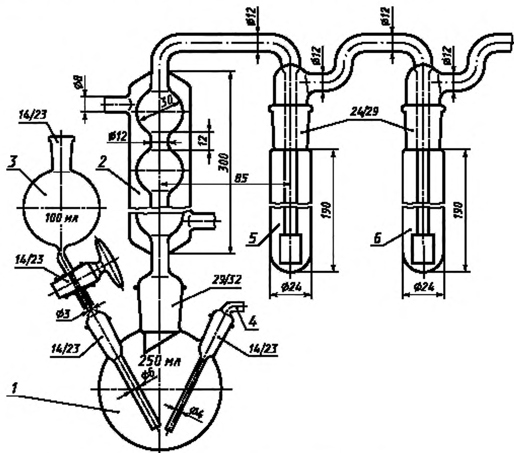
1 — дистилляционная колба; 2 — обратный холодильник; 3 — капельная воронка; 4 — подводящая трубка, 5 и 6 — газопоглощающие устройства
