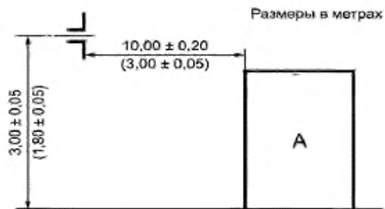
а) Положение симметричной дипольной антенны для измерения вертикальной компоненты излучения
