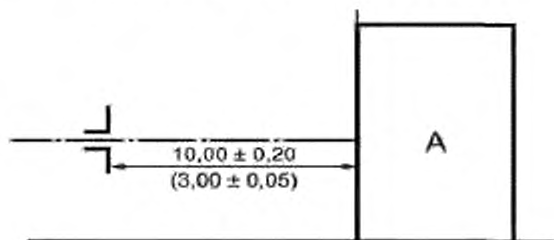
б) Положение симметричной вибраторной антенны для измерения горизонтальной компоненты излучения
