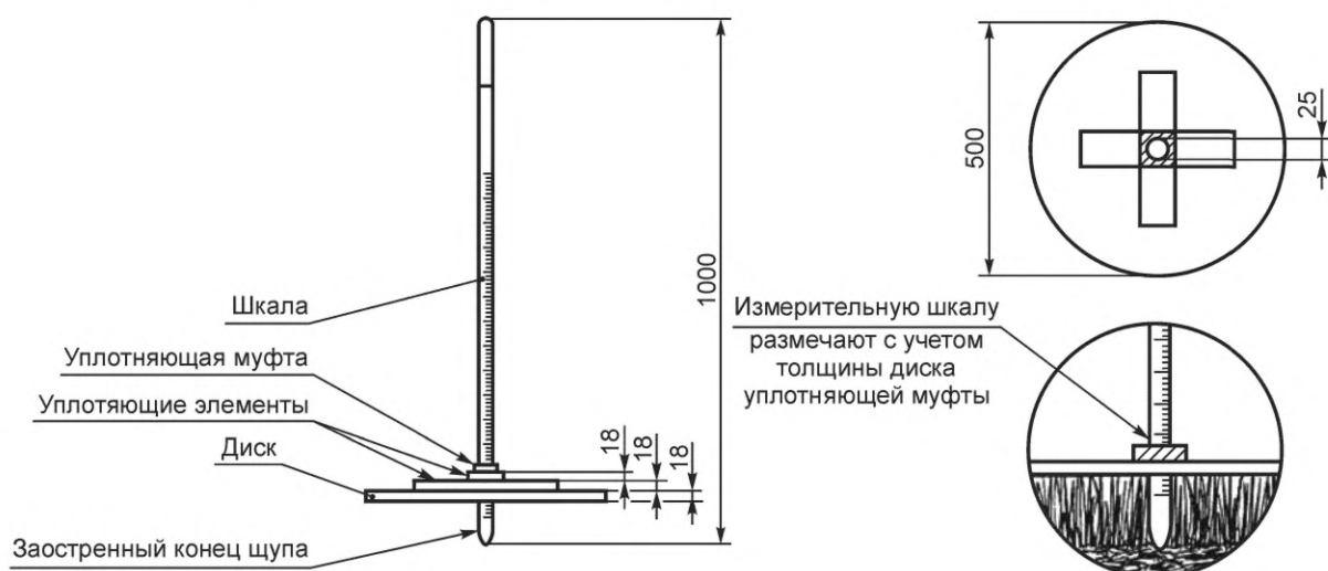
Рисунок 2 — Измерительный диск
