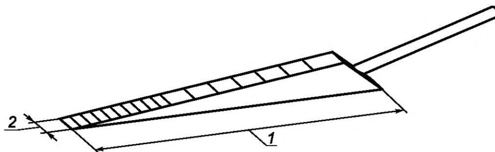
Рисунок 10 — Измерительный клин
