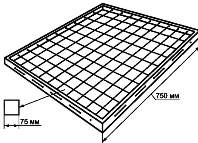
Рисунок 3 — Рама для измерения плотности травяного покрова
