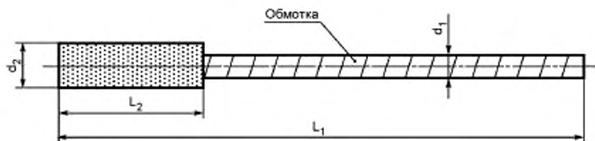
Рисунок Л.2 — Композитная гибкая связь с цилиндрическим лесчатым анкерным участком
