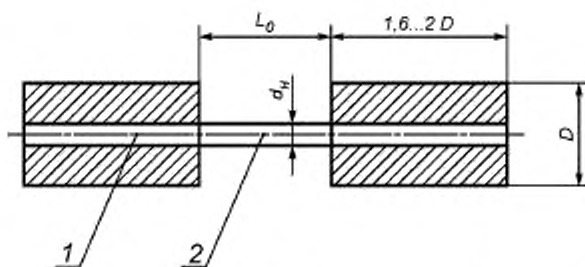
1 — испытательная муфта; 2 — отрезок композитной гибкой связи
