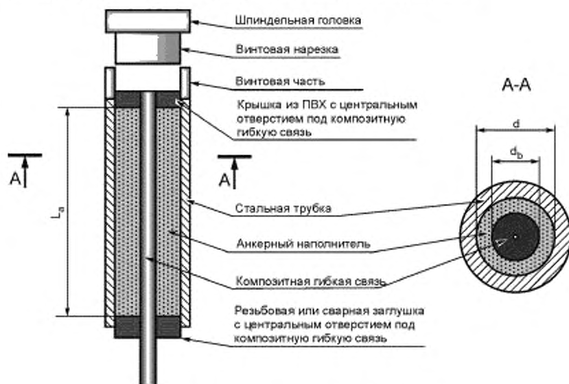
Рисунок Б.1 Конструкция испытательных муфт
