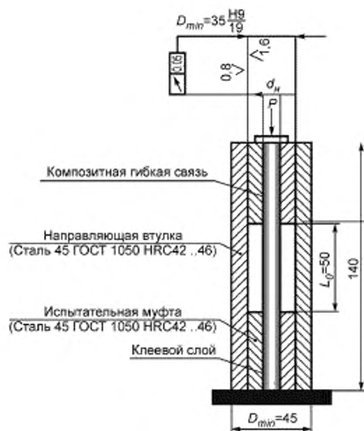
Рисунок В.1 — Конструкция приспособления для испытания образцов
