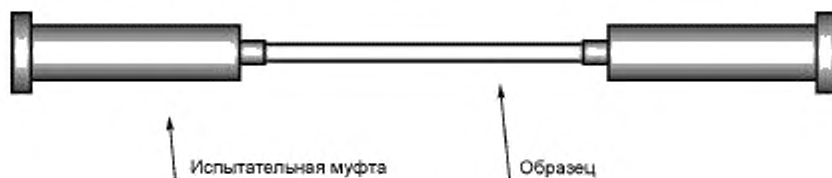
Рисунок Б.2 — Общий вид образцов для испытания
