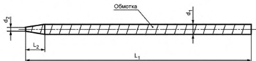
Рисунок Л.3 — Композитная гибкая связь с выделенным анкерным участком под анкерную гильзу
