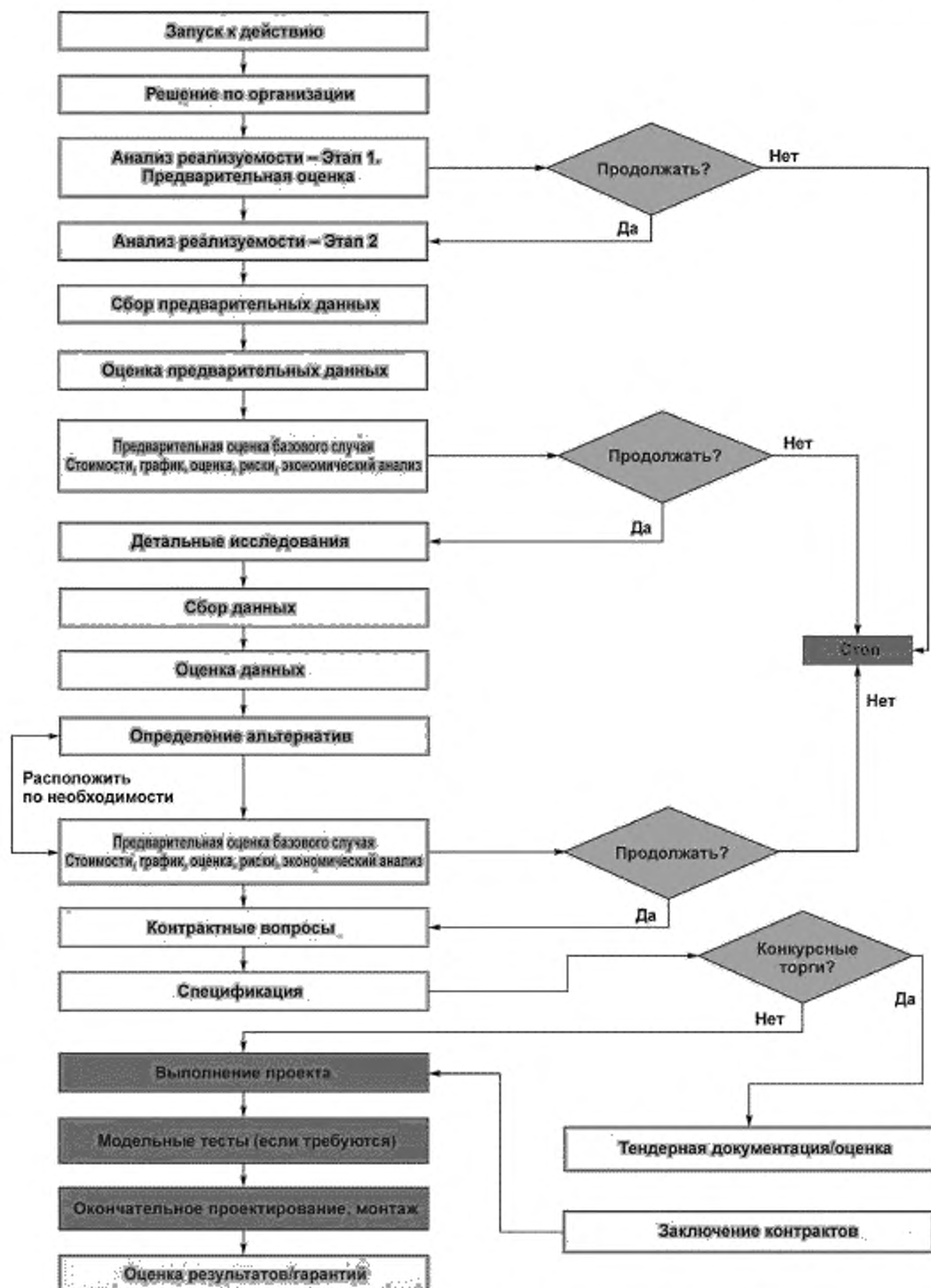
Рисунок 1 — Блок-схема, описывающая этапы проведения ремонта
