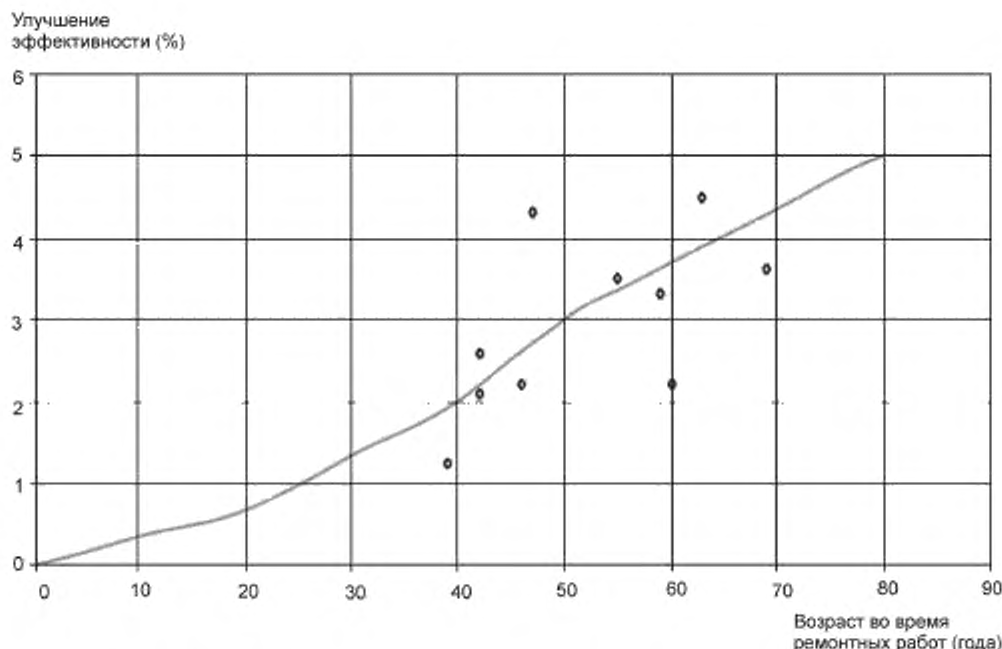
Рисунок 7b — Потенциальные усовершенствования для ремонта турбины Каплана
