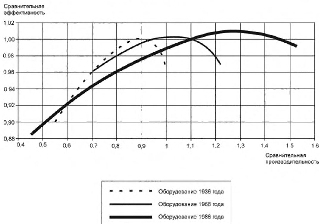
Рисунок 3 — Сравнительная эффективность по сравнению с сравнительной производительностью — первоначальные и новые рабочие колеса
