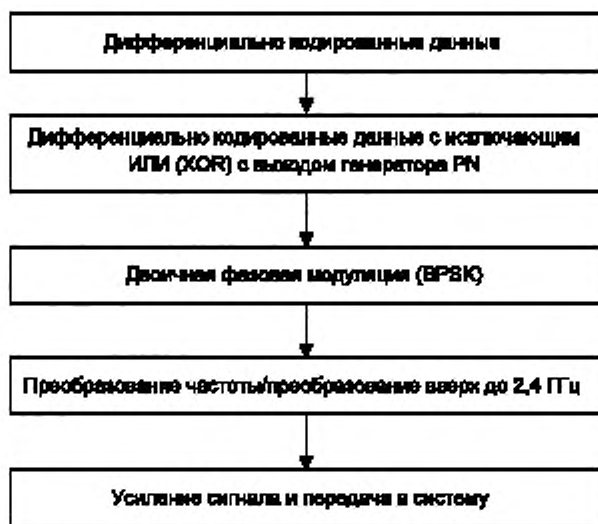
Рисунок 6 — Процесс кодирования и передачи данных передатчика
