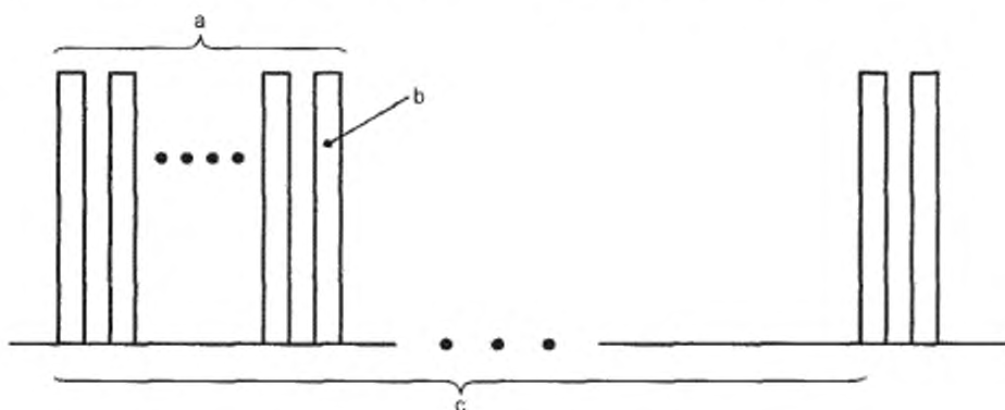
а — пачка, содержащая N субпачек; б — субпачка; с — интервал пачки
