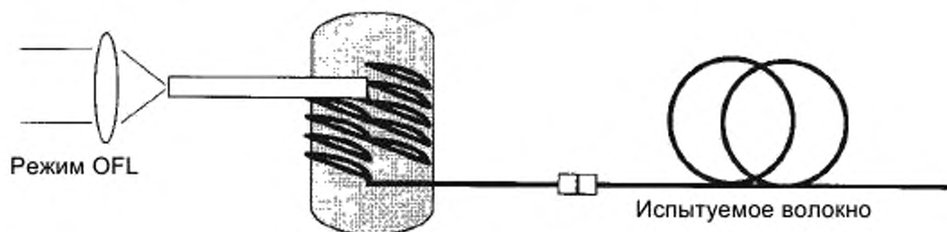
Рисунок 1 – Модовый фильтр, намотанный на оправку
