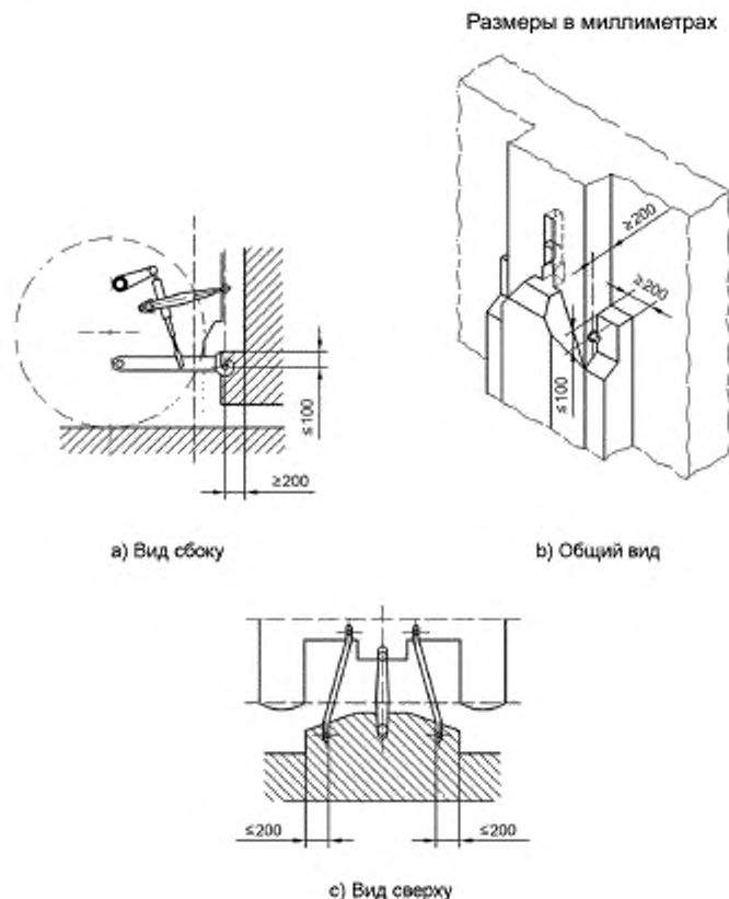
Рисунок 2 — Зона сцепления
