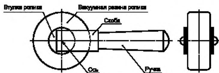
Рисунок Г.3 — Ролик для прикатывания ТЭ
