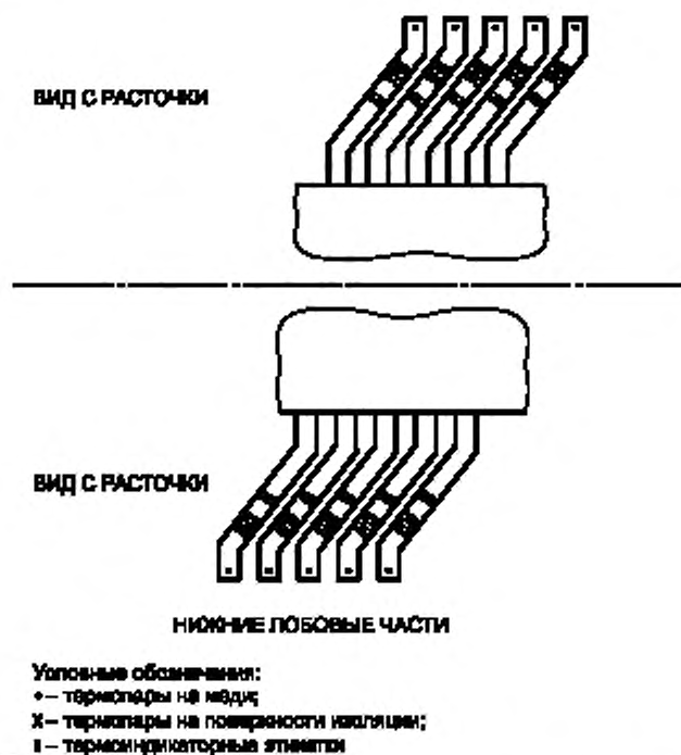
Рисунок Г.2 — Схема установки термодар и ТЭ на лобовых частях обмотки статора гидрогенератора
