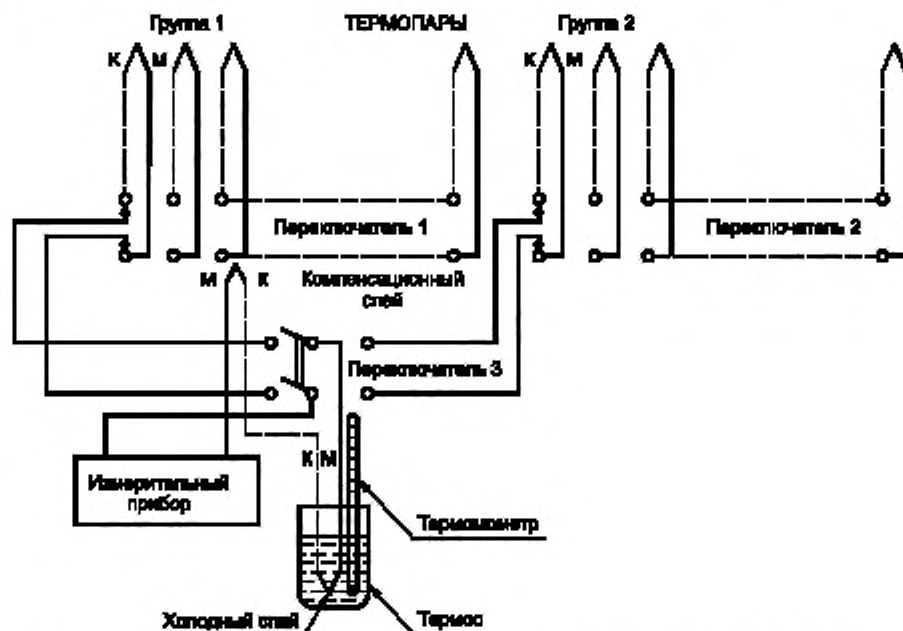
Рисунок Г.1 — Схема измерений температуры паяк обмотки статора гидрогенератора при помощи термомпар
