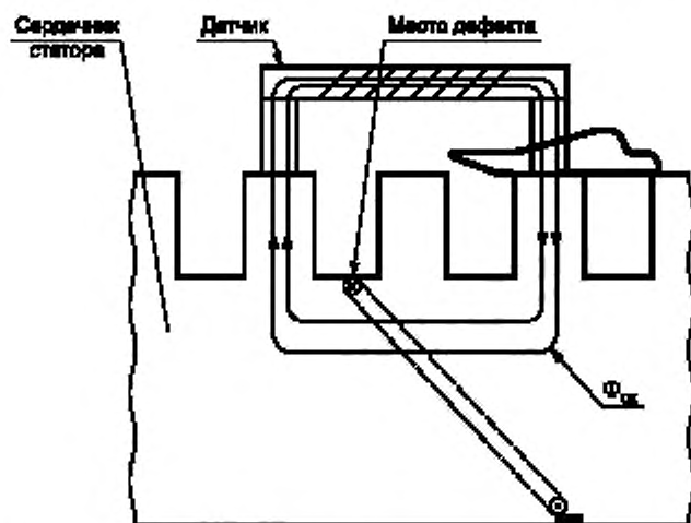
Рисунок К.2 — Способ установки датчика на зубцы сердечника статора в месте дефекта
