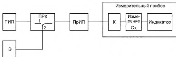
Рисунок Б.4 — Структурная схема калибровки ИК поэлементным методом для индивидуального измерительного прибора
