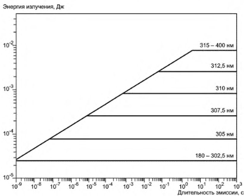
Рисунок В.4 — ПДЭ для излучающего ультрафиолетового лазера класса 1 с длительностью эмиссии от 10^{-9} до 10^3 с для определенных длин волн
