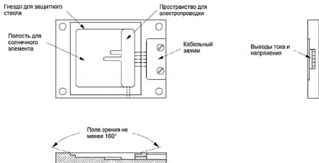
Рисунок 2 – Корпусирование одиночного солнечного элемента.
