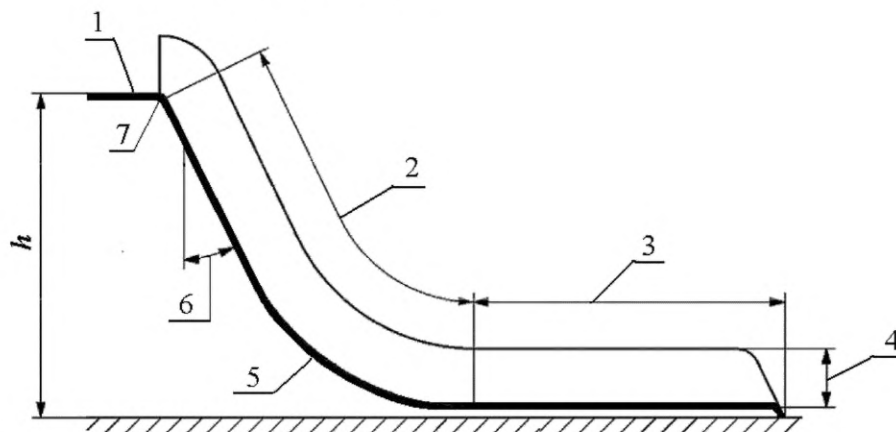
1 — стартовый участок; 2 — участок скольжения; 3 — конечный участок; 4 — бортики; 5 — радиусный элемент нижней части участка скольжения; 6 — угол наклона участка скольжения к вертикали; 7 — радиусный элемент верхней части участка скольжения (не менее 100 мм); h — высота горки
