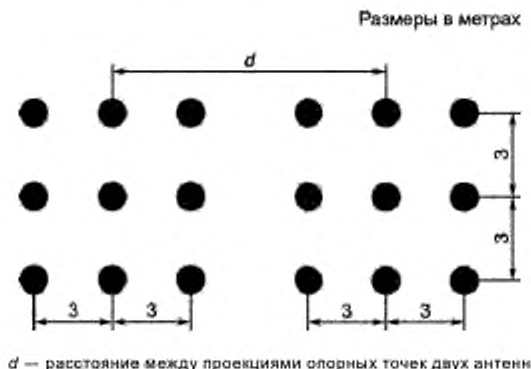
Рисунок 32 — Размещение парных испытательных точек для всех испытательных расстояний
