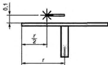
Рисунок 15 — Позиция антенны над установочным столом (вид сбоку)
