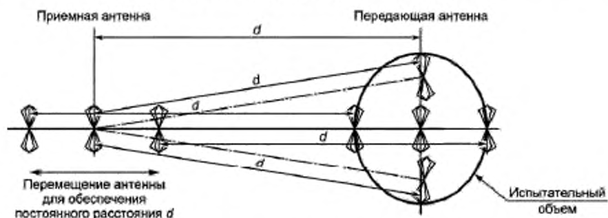
Рисунок 36 — Типовые позиции антенн для OATS с укрытием от атмосферных воздействий и SAC. Измерения для валидации при горизонтальной поляризации
