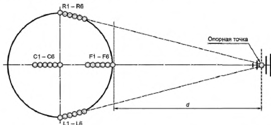
Рисунок 20 — Позиции при измерении S_{VSWR} в горизонтальной плоскости (см. 8.3.3.2.2)
