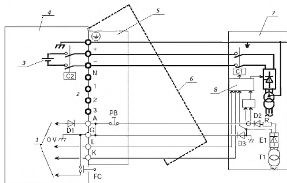
1 — к электронному узлу управления; 2 — присутствие переносной розетки; 3 — главная батарея; 4 — ЭТ; 5 — переносная розетка; 6 — откидная дверь; 7 — специализированное оборудование питания.
