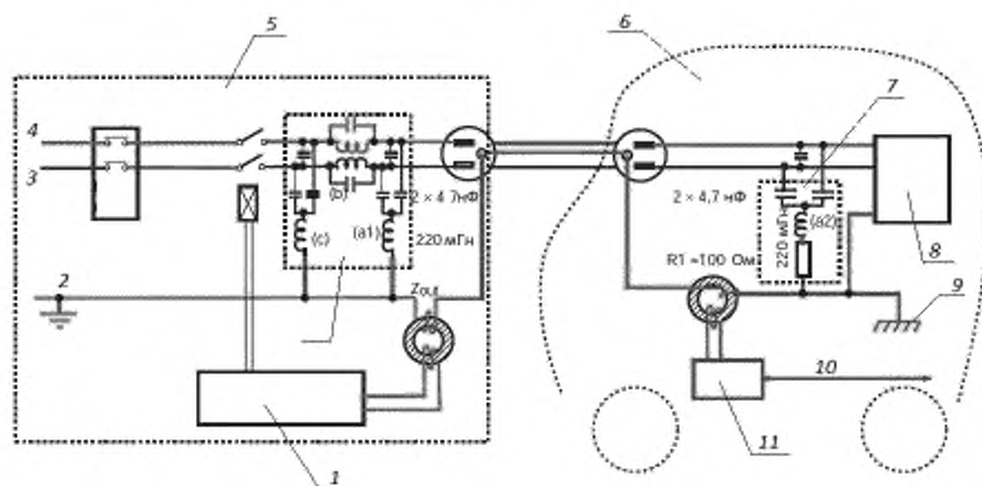
1 — модем с командным реле; 2 — земля; 3 — фильтр; 4 — нейтраль; 5 — стационарная силовая розетка; 6 — ЭТ или ПГДЭТ; 7 — VЧ фильтр; 8 — зарядное устройство ЭТ; 9 — шасси ЭТ; 10 — команда ЭТ; 11 — модем
