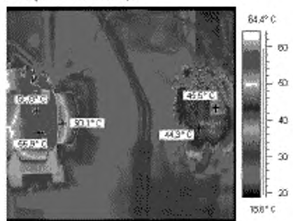
Рисунок С.7 – Корпуса подшипников шестерни привода мельницы
