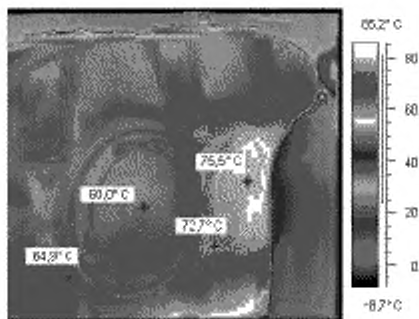
Рисунок С.5 – Редуктор со стороны двигателя
