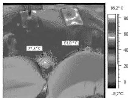
Рисунок С.6 – Редуктор со стороны мельницы
