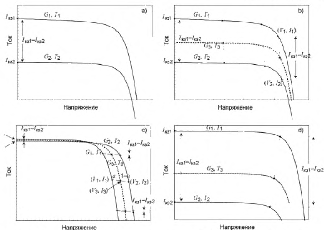
Рисунок 1 – Пример коррекции ВАХ с применением уравнений (6) и (7). Рисунки (а) и (б) изображают коррекцию по энергетической освещенности, Рисунок (с) изображает коррекцию по температуре и Рисунок (д) – коррекцию одновременно по энергетической освещенности и температуре.
