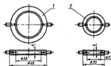
1 — кольцо для больших пробирок; 2 — кольцо для малых пробирок
