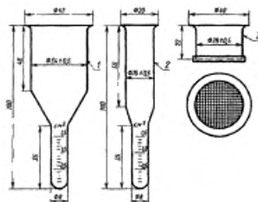
1 — большая пробирка; 2 — малая пробирка; 3 — стакан с ситом
