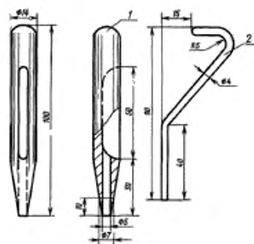
1 — пробоотборник; 2 — паршень
