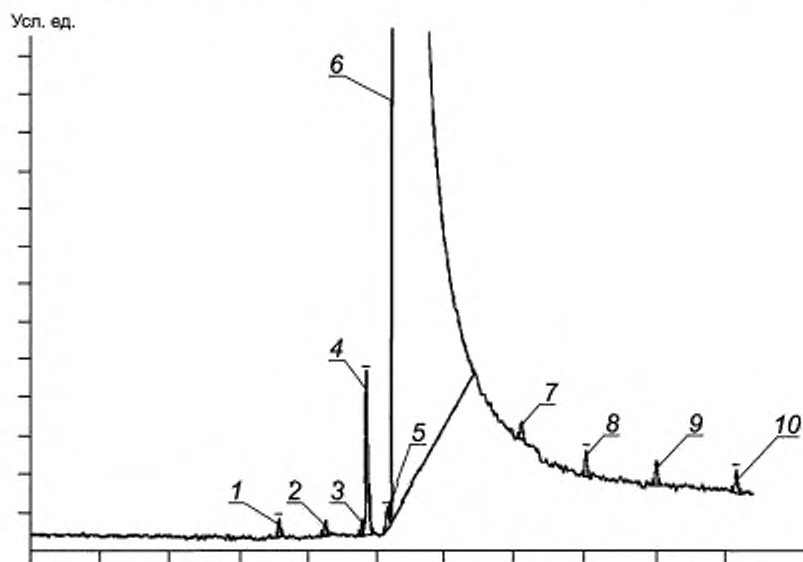
1 — уксусный альдегид; 2 — метилацетат; 3 — этилацетат; 4 — метанол; 5 — пропанол-2; 6 — этанол; 7 — пропанол-1; 8 — изобутанол; 9 — бутанол-1, 10 — изопентанол
