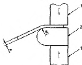
1 Зажим 2 Пуансон Рисунок 3
