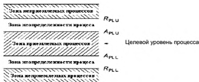
Рисунок 1—Границы требований к процессу: верхняя и нижняя линии APL и RPL, зоны приемлемости и неприемлемости и неопределенности процесса
