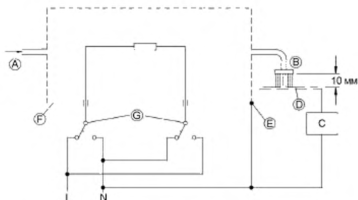
А — входная трубка; В — распылительная головка; С — цель по МЭК 60990 (рисунок 4); D — металлическая сетка; E — зажим заземления; F — корпус водонагревателя; G — переключатель; L — фаза; N — нейтраль
