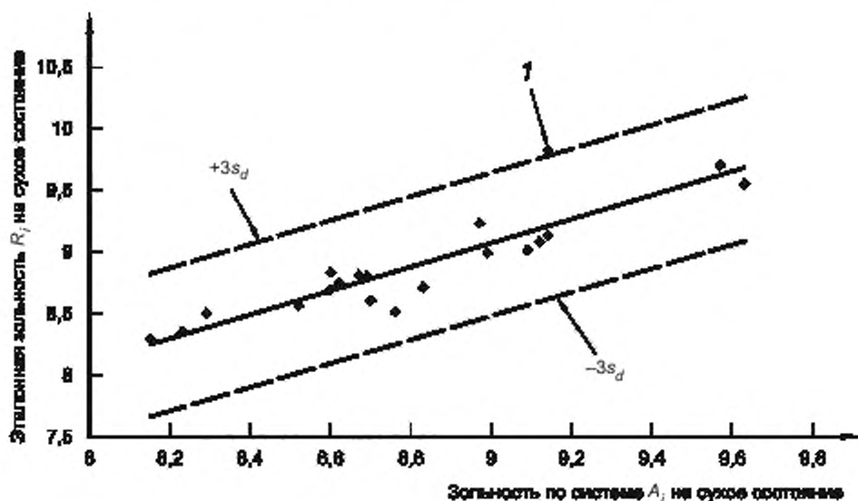
Рисунок A.1 — График разброса контрольных и системных значений
