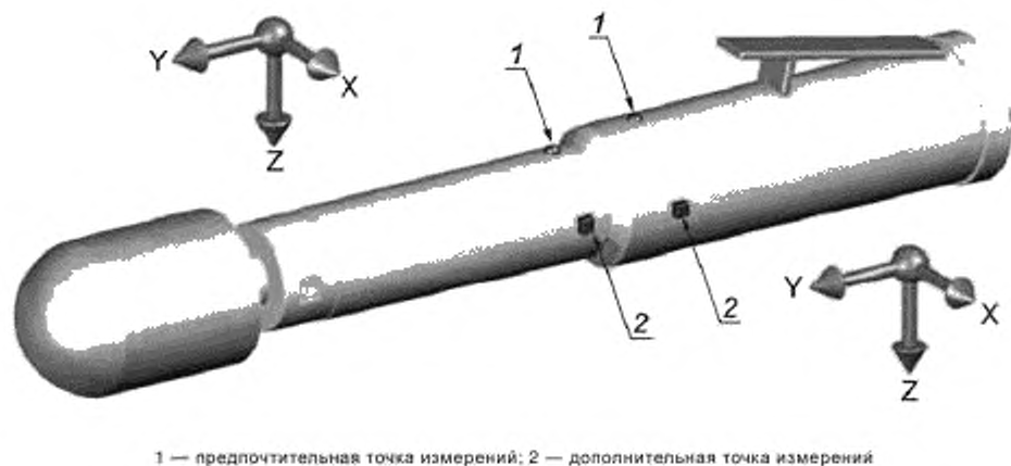
Рисунок 5 — Точки и направления измерений для прямой шлифовальной машины с шлифовальной головкой типа 18R
