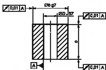
Рисунок С.5 — Геометрические размеры и допуски на изготовление промежуточной втулки для испытательных кругов типа 1
