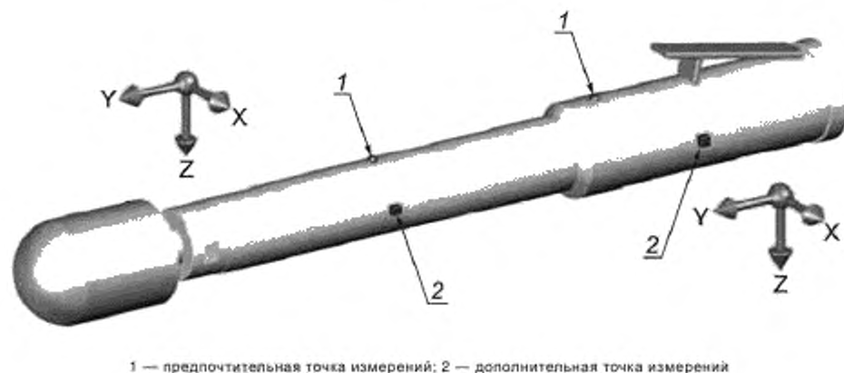
Рисунок 6 — Точки и направления измерений для прямой шлифовальной машины с шлифовальной головкой типа 18R и удлиненной рукояткой
