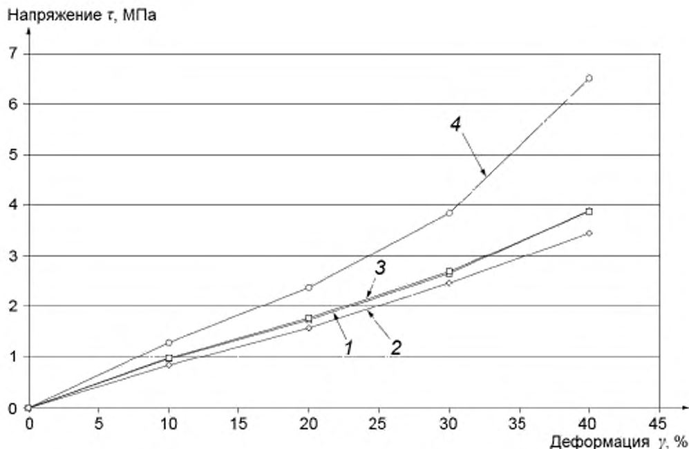
1, 2, 3, 4 – первый, второй, третий и четвертый образцы соответственно Рисунок А.2 – Статические упругопрочностные свойства при сжатии приклеенных образцов для испытания (напряжения приведены без поправок)
