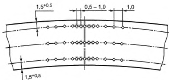
е — Труба HFW
