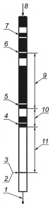
1 — нижняя часть; 2 — фронт элюирования; 3 — чистая жидкость; 4 — первая интенсивная желтая флуоресценция; 5 — первая интенсивная голубая флуоресценция; 6 — красно-коричневое кольцо; 7 — дополнительное красное кольцо; 8 — верхняя часть; 9 — зона ароматики; 10 — зона олефинов; 11 — зона насыщенных углеводородов
