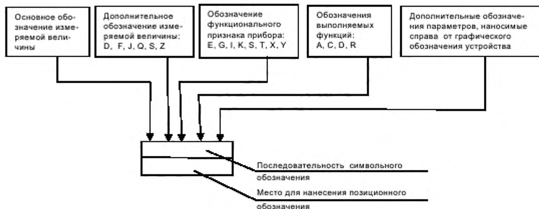
Рисунок 1 — Принцип построения условного обозначения прибора
